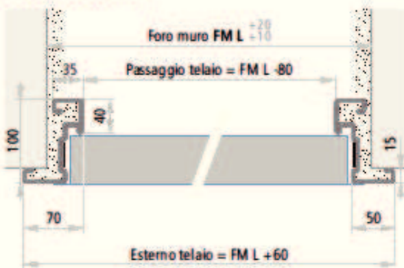
Porta ad un'anta Sezione orizzontale
