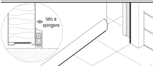
Figura G VERSIONE CON GUARNIZIONE SOTTOPORTA (Combo S200; Combo S200V; Combo dB Sa; Combo dB Sa/V; Combo dB; Combo dB/V)
