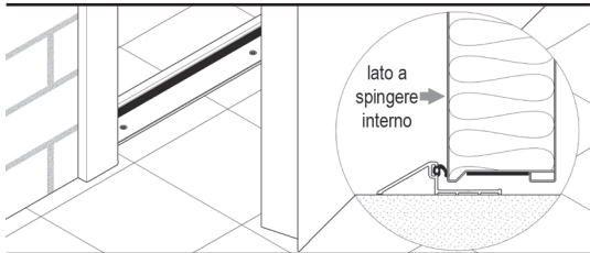
Figura F VERSIONE CON SOGLIA FISSA INFERIORE
