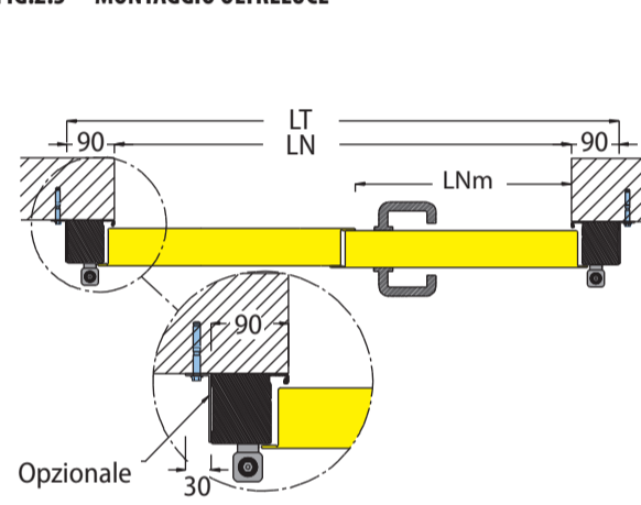
FIG.2.3 MONTAGGIO OLTRELUCE
