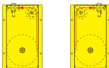
FIG. 6.5 POSIZIONAMENTO E VERIFICA CHIUDIPIORTA
