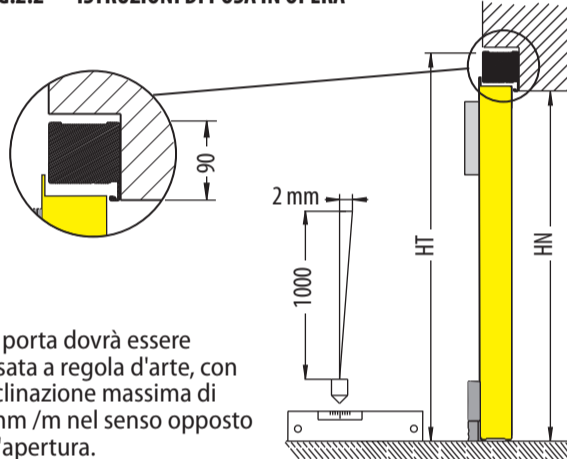
FIG.2.2 ISTRUZIONI DI POSA IN OPERA
