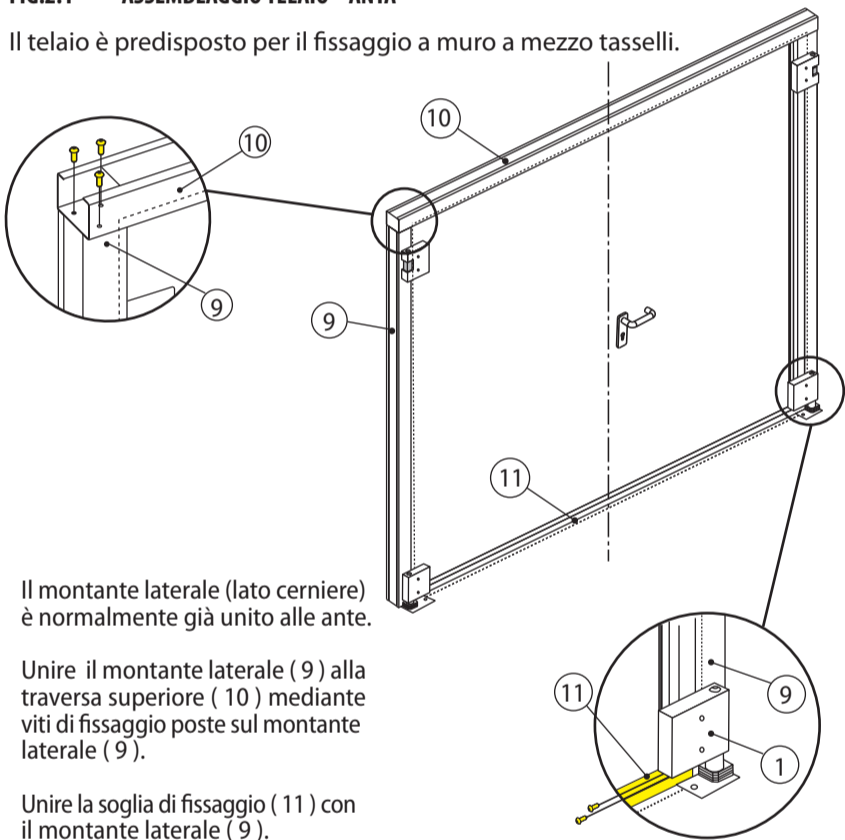
FIG.2.1 ASSEMBLAGGIO TELAIO - ANTA
