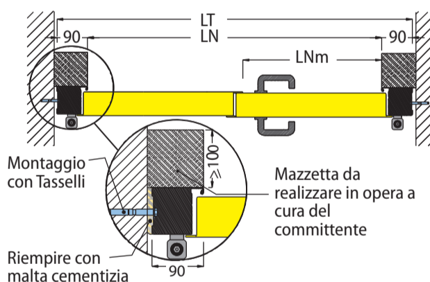
FIG.2.5 MONTAGGIO IN CORRIDOIO O IN LUCE
