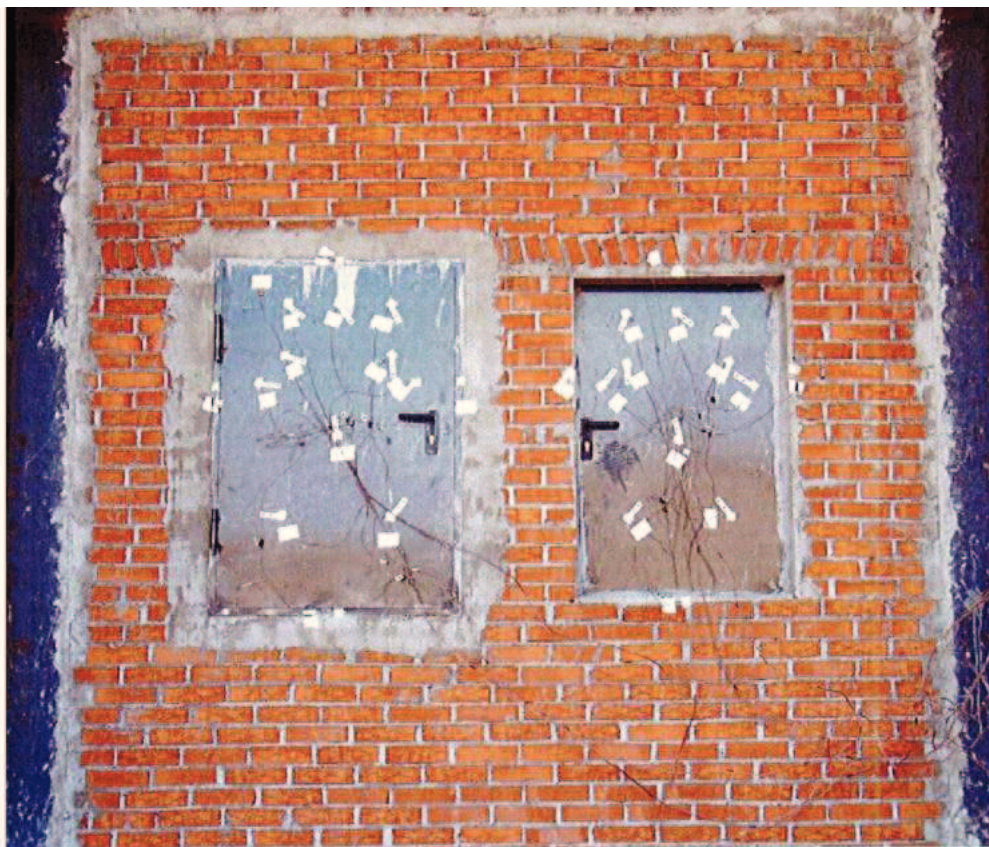
Foto 2. Lato non esposto al fuoco del manufatto prima della prova
